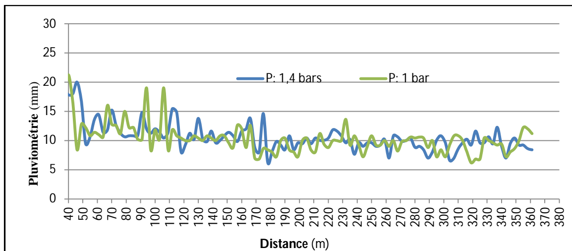
Figure 8.- Effet de la variation de la pression de fonctionnement sur la répartition pluviométrique sous le pivot (LINDSAY ZIMMATIC) avec vitesse du vent (3-5 m/s)
