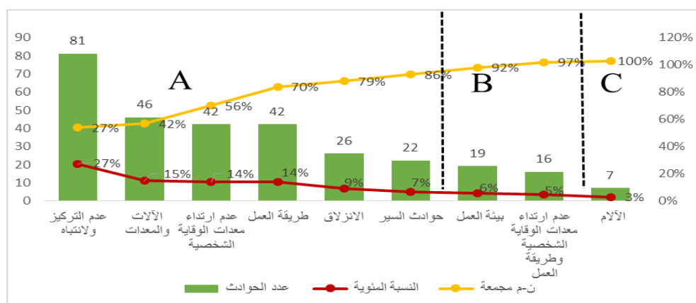
الشكل (9) تصنيف أسباب الحوادث المهنية لمجموع العوامل باستخدام طريقة ABC بالنسبة لمؤشر عدد الحوادث
