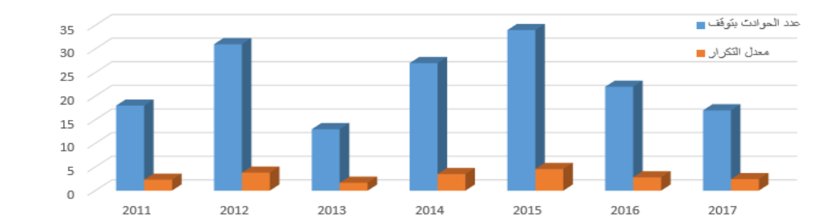
الشكل (6) يوضح تطور معدل التكرار بالتزامن مع تطور حوادث العمل بالتوقف
